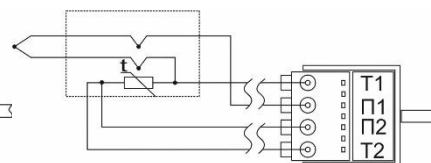
Схема подключения ТП с компенсационным ТС
