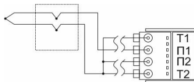
Схема подключения ТП без компенсационного ТС
