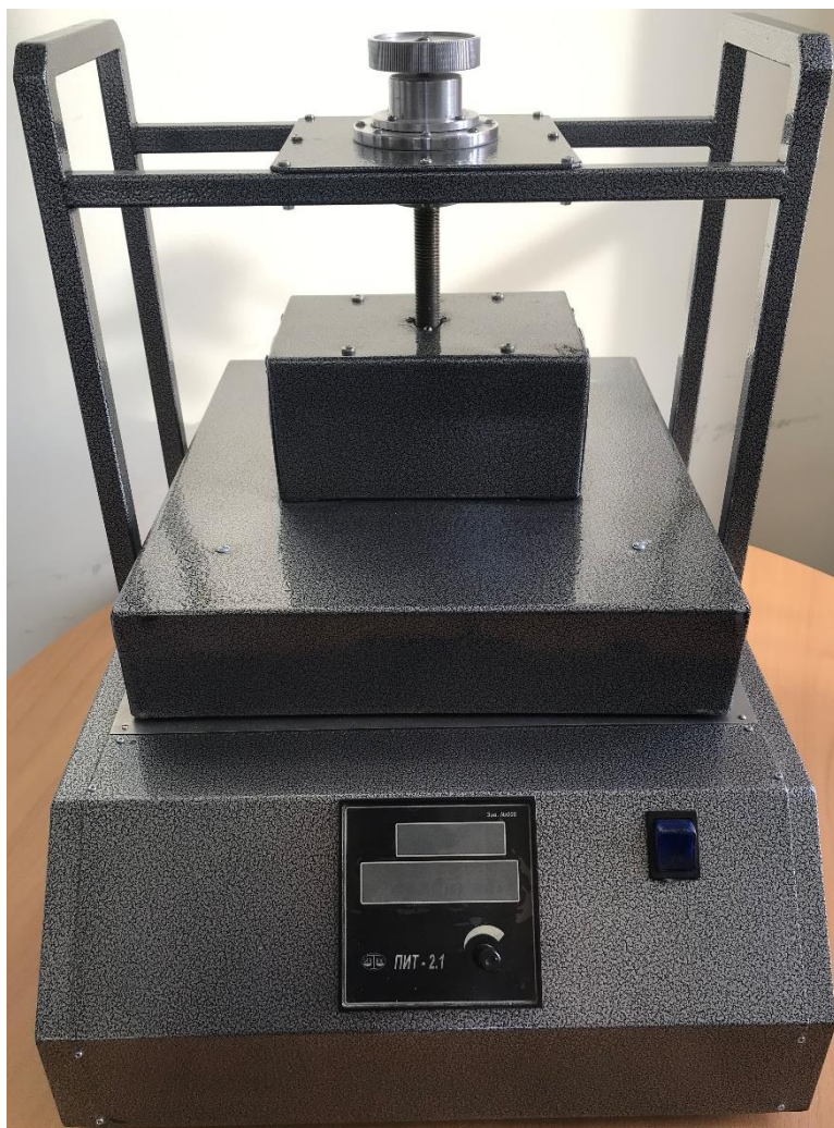
Рисунок 1 – Общий вид прибора для измерения теплопроводности ПИТ-2.1
