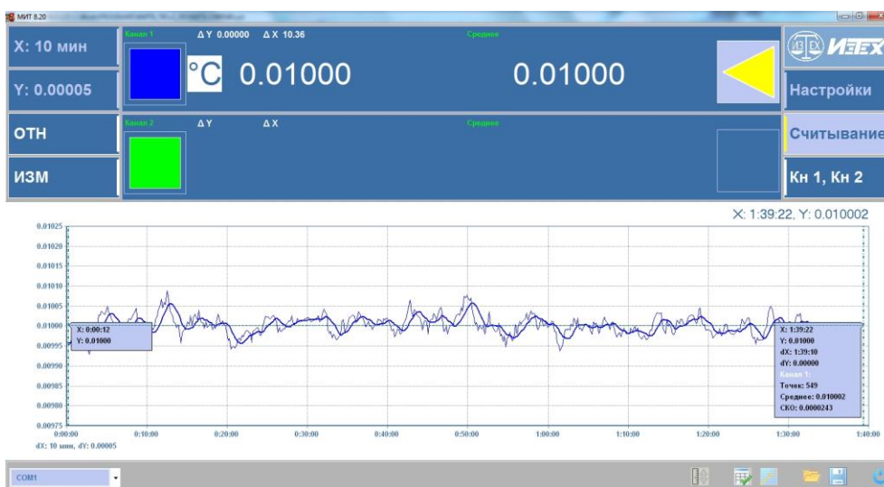
График температурного хода в ампуле тройной точки воды АТТВ-1, измеренного при помощи ПТС-10М (ток питания 1мА) и МИТ 8.20. СКО измерений составило 0.024мК.
