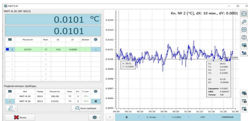
График температурного хода в ампуле тройной точки воды АТВВ-1, измеренного при помощи ПТС-10М (ток питания 1мА) и МИТ 8.30. СКО измерений составило 0.047мК.
