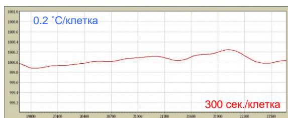
График хода температуры в калибраторе температуры КТ-3 с регулятором РТП-8.3 в зависимости от времени. ТП (ТНН) в качестве датчика температуры.
